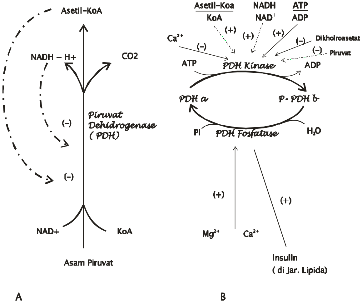
Gambar 6. Kontrol Piruvat Dehidrogenase A.Kontrol dengan hambatan hasil reaksi B.Kontrol dengan perubahan aktif atau tidak aktif
